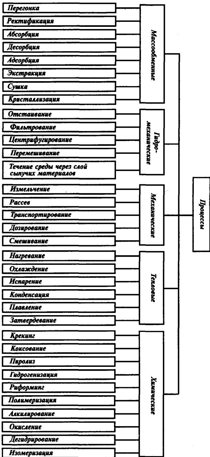
Рис. В-1. Схема классификации основных (типных) процессов нефтегазопереработки и нефтехимии
